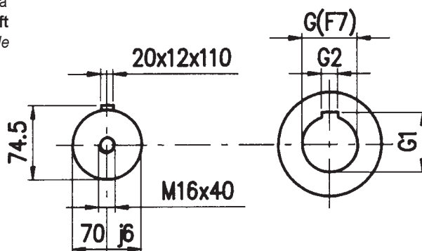
Albero entrata Input shaft Antriebswelle
