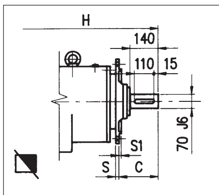
Albero uscita Output shaft Abtriebswelle
